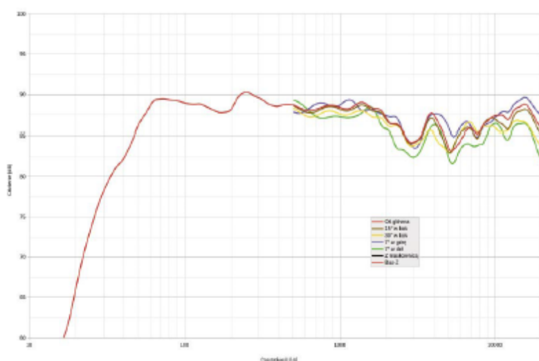
Rys. 1. Charakterystyka przetwarzania na różnych osiach, powyżej 500 Hz.
